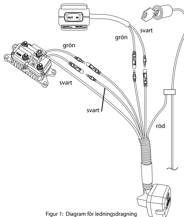
Figur 1: Diagram för ledningsdragning
